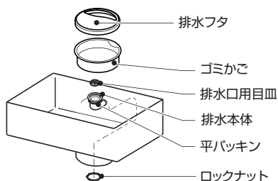
(SPシンク用)
