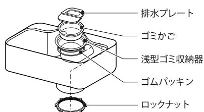
(Dシンク用)
