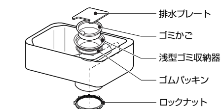
(Vシンク用)
