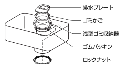
(Nシンク用)
