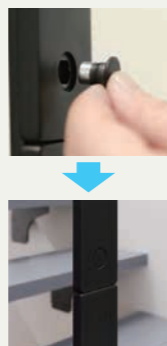
手摺手前部分の接合部は座彫りしており、フラットな形状になるよう工夫。
