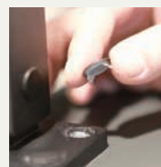
踏板の水平面だけでなく垂直面もビス留めし、より強固に固定することで安全性を向上。
